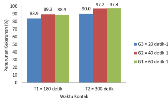
Gambar 4. Persentase Penurunan Kekeruhan
